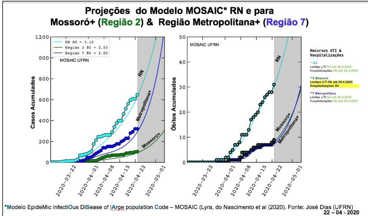
Figura 6 - Número de casos e óbitos acumulados por covid-19 e projeções do modelo matemático para a 2a. Região de Saúde (Mossoró) e 7a. Região de Saúde (Natal).
